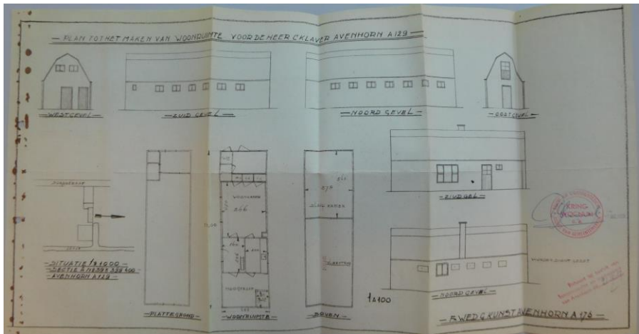
Verbouwingstekening van de schuur uit 1929 tot woning
